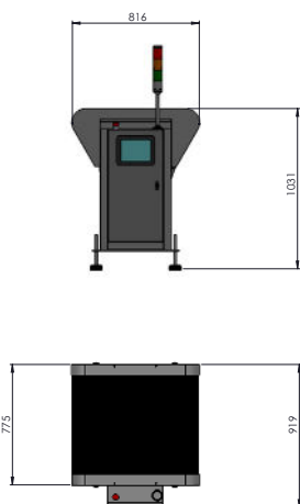
Erizo 60
