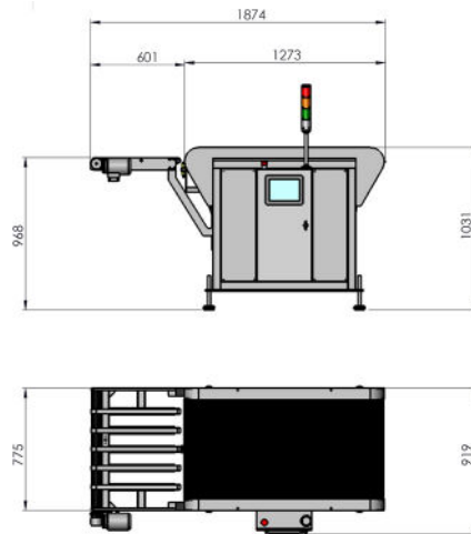
Erizo 100 + Conveyor
