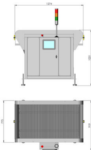
Erizo 100
